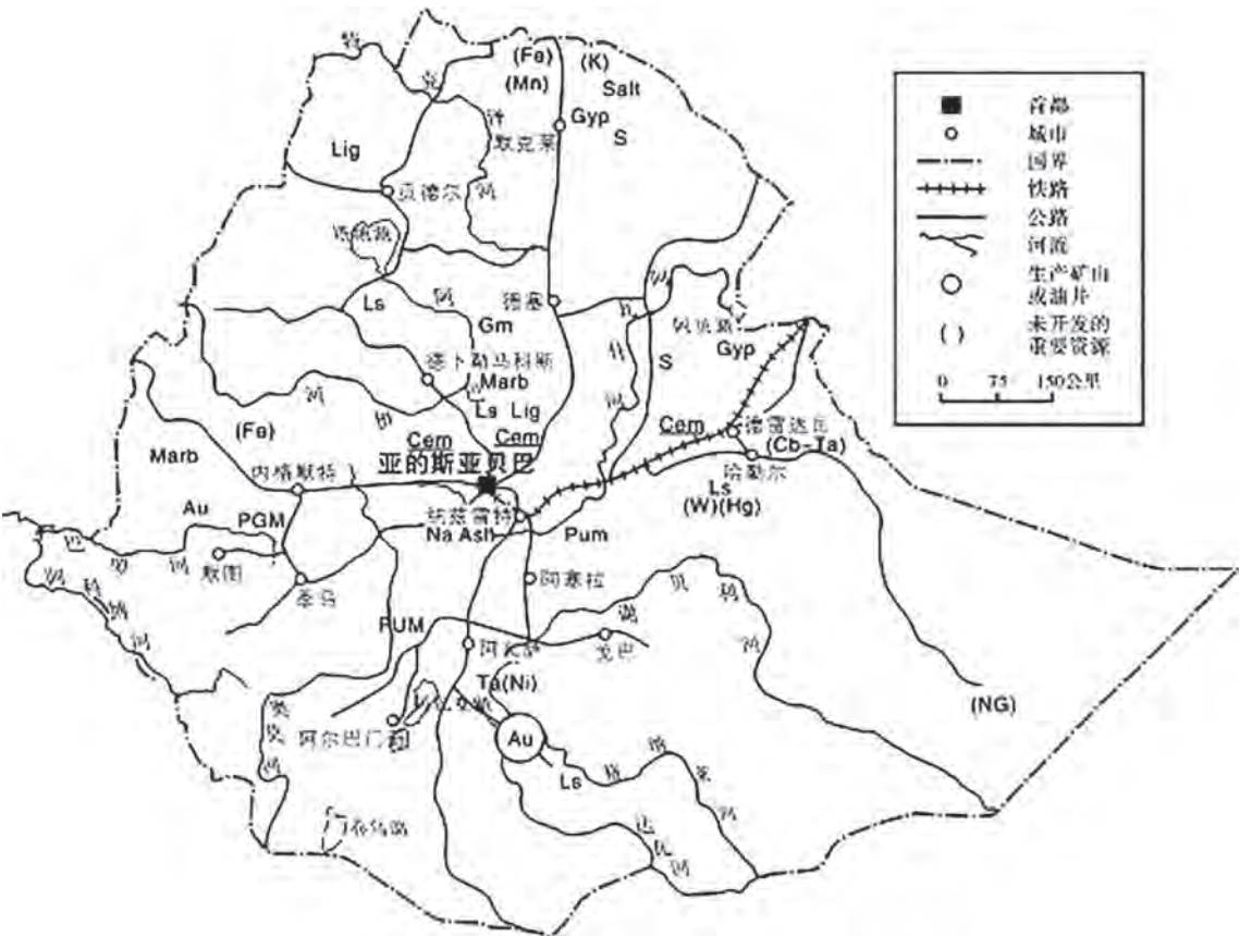
图 3-8 埃塞矿产资源分布 ③
